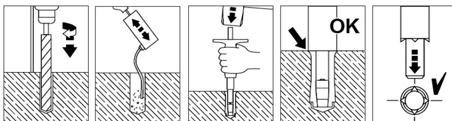
Fig. 4-2: Istruzioni per l'inserimento dei tasselli (Fonte: Ditta Hilti)
