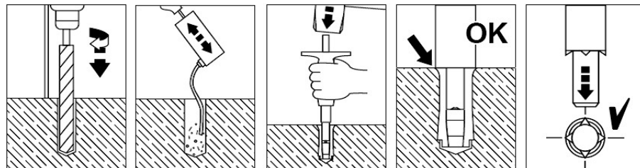
Afb. 4-2: Handleiding voor het plaatsen van pluggen (Bron: Hilti)
