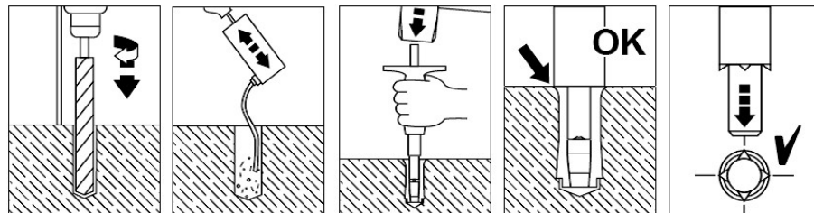
Fig. 4-2: Instructions pour la pose des chevilles (Source : Sté Hilti)
