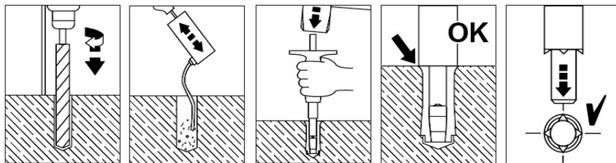
Abb. 4-2: Anleitung zum Setzen der Dübel (Quelle: Fa. Hilti)
