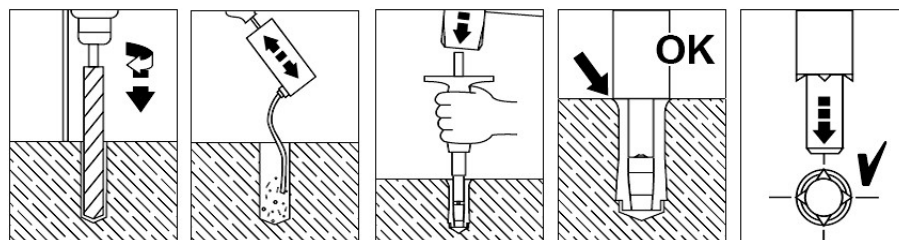
Fig. 4-2: Instruções sobre a colocação das buchas (Fonte: Empresa Hilti)
