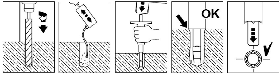
Fig. 4-2: Instrucciones de colocación de los tacos (Proveedor: Hilti)
