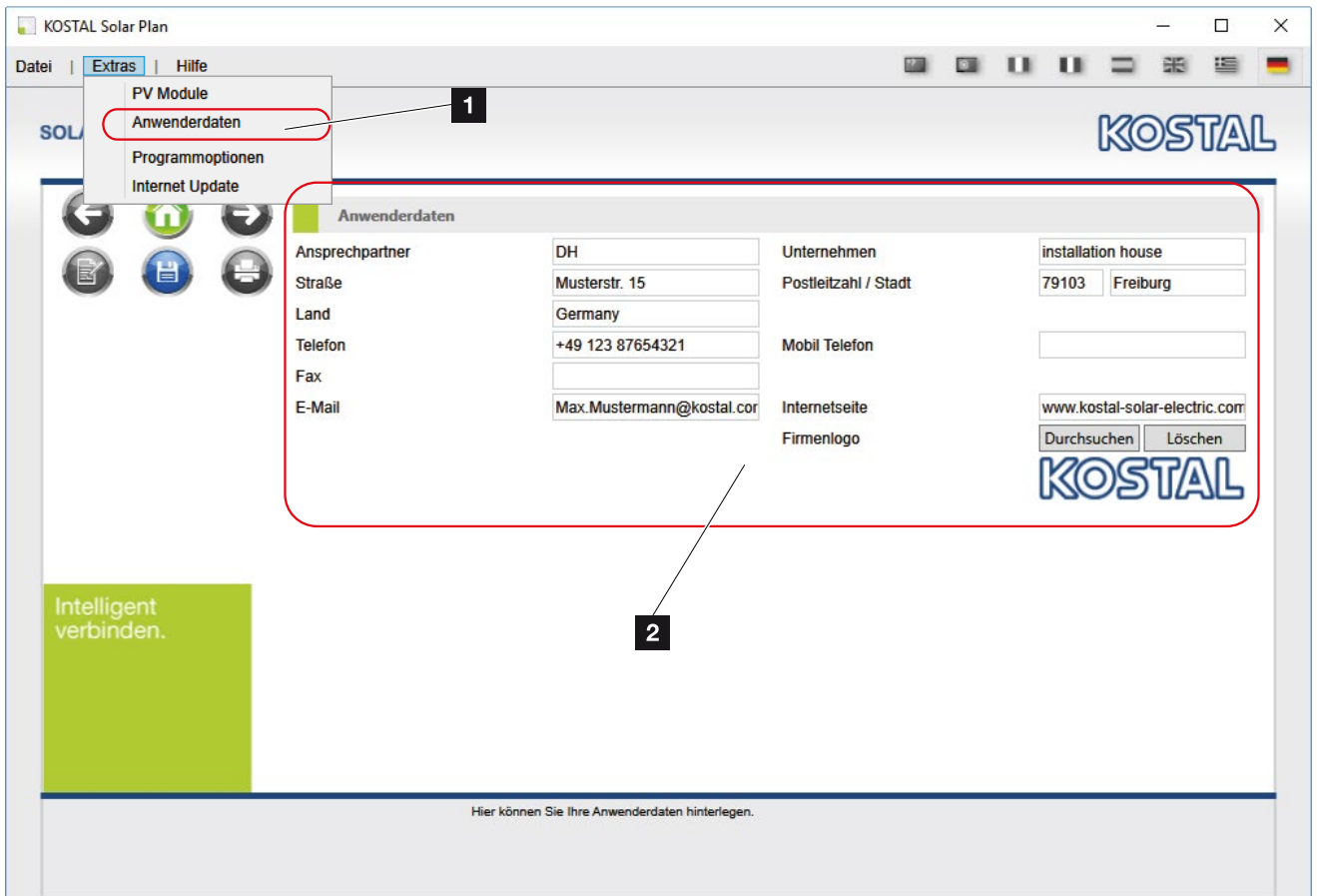
Abb. 8: Anwenderdaten
