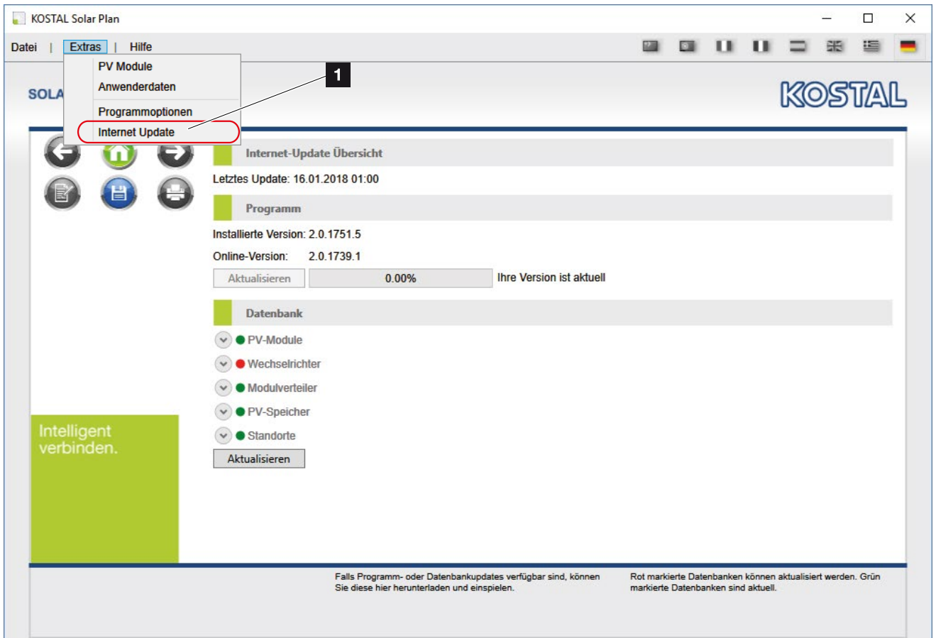
Abb. 11: Update
