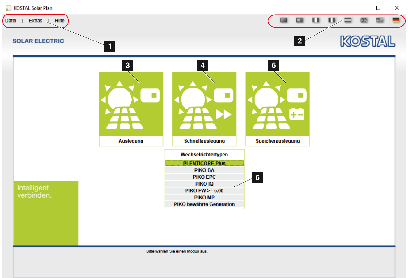
Abb. 7: Startbildschirm
