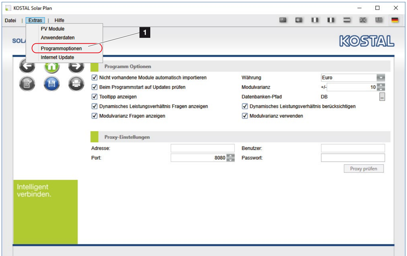
Abb. 10: Programmoptionen
