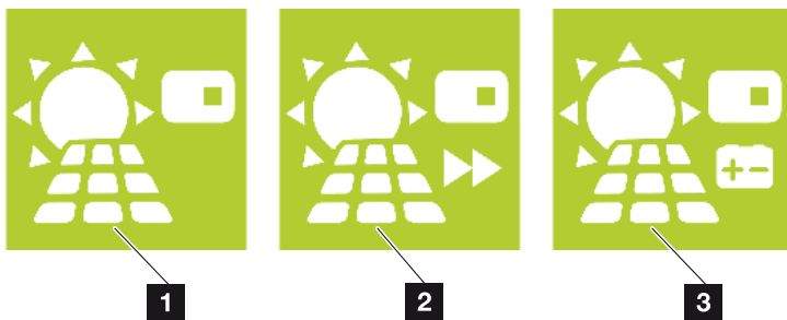
Abb. 12: Planungsauswahl
