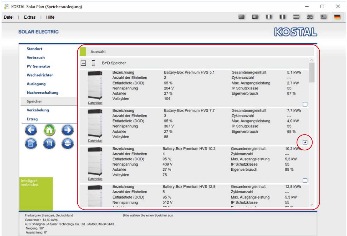
Abb. 30: Batteriespeicher auswählen
