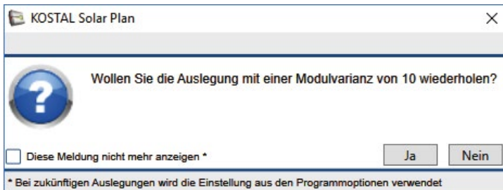
Abb. 20: Frage - Modulvarianz
