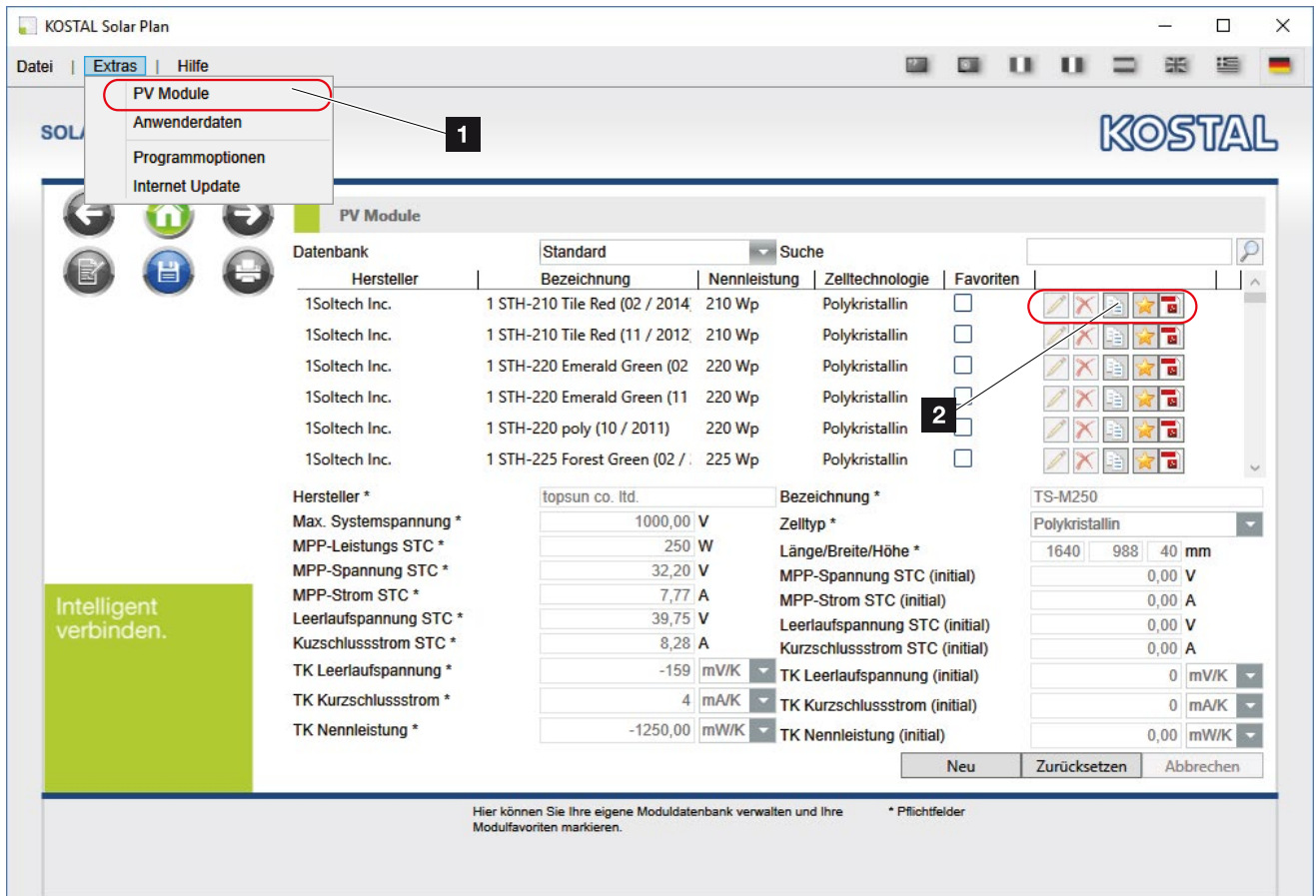
Abb. 9: PV-Moduldatenbank
