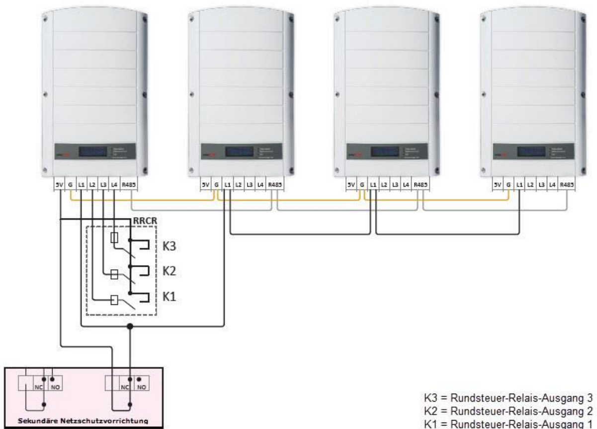
Abbildung 4: Anlage mit mehreren Wechselrichtern mit RRCR
