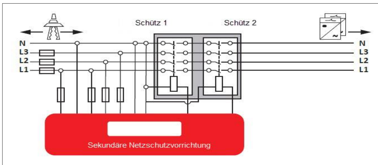
Abbildung 1: Sekundäre Netzschutzvorrichtung
