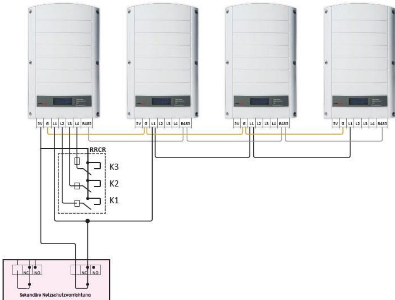
Abbildung 6: Drei-Relais-RRCR und eine AC-Relaissteuerung
